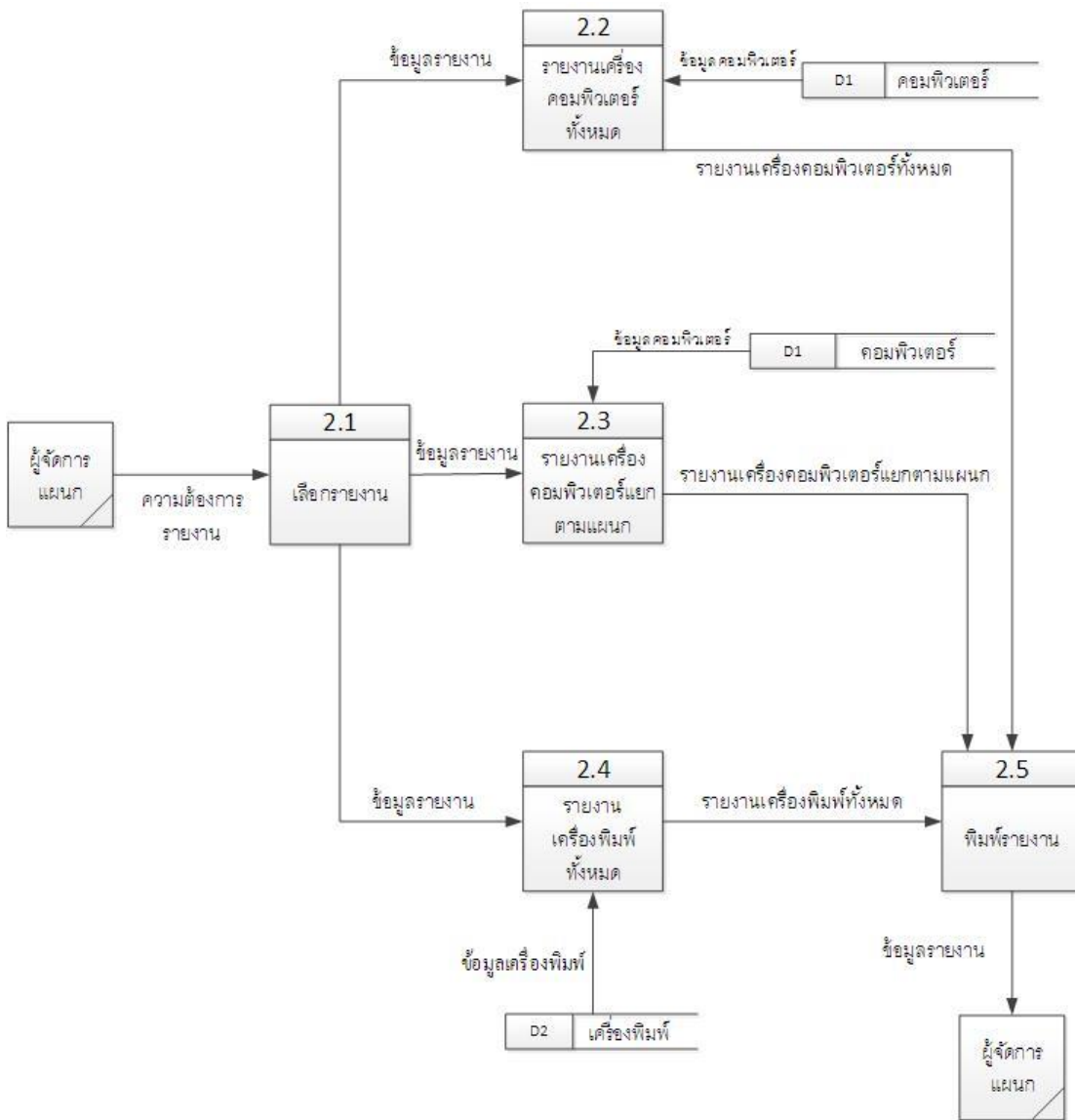
รูปที่ ก.6 Data Flow Diagram Level 1 ของ Process 2 : ออกรายงาน
