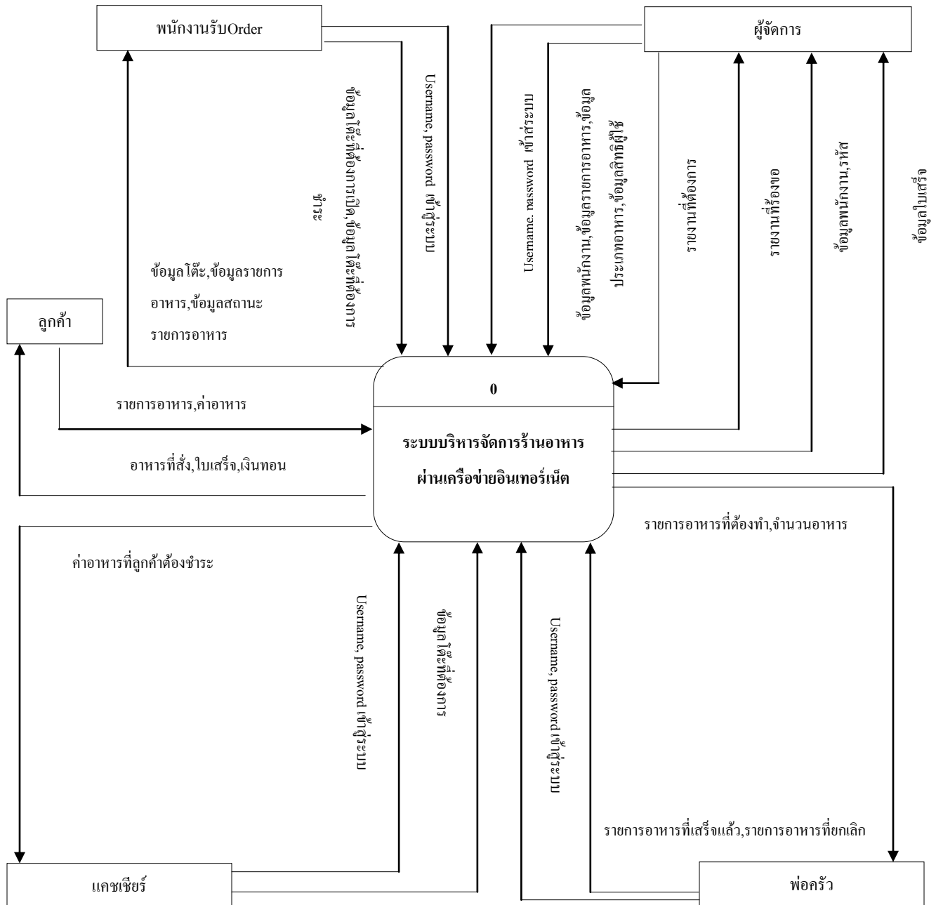
รูปที่ 3.2 แสดงแผนภาพ Context Diagram ของระบบบริหารจัดการร้านอาหารผ่านเครือข่ายอินเทอร์เน็ต
