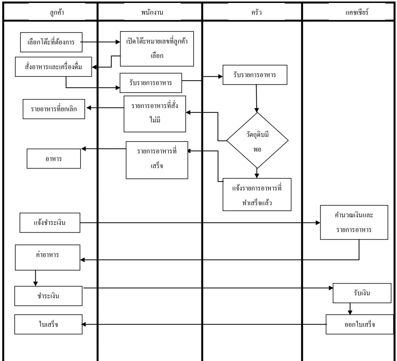
รูปที่ 3.1 แผนผังการทำงานของระบบงานใหม่ (Work Flow Diagram)
