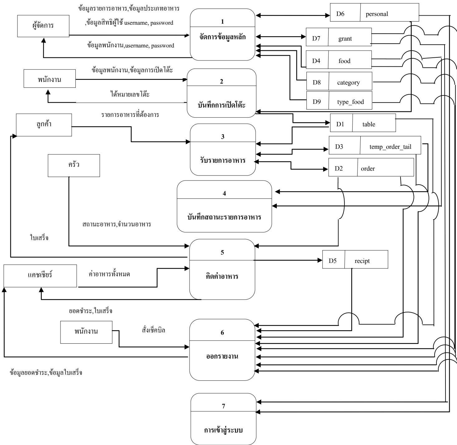
รูปที่ 3.2 แสดงแผนภาพ Data Flow Diagram (DFD Level-1)ของระบบบริหารจัดการ
