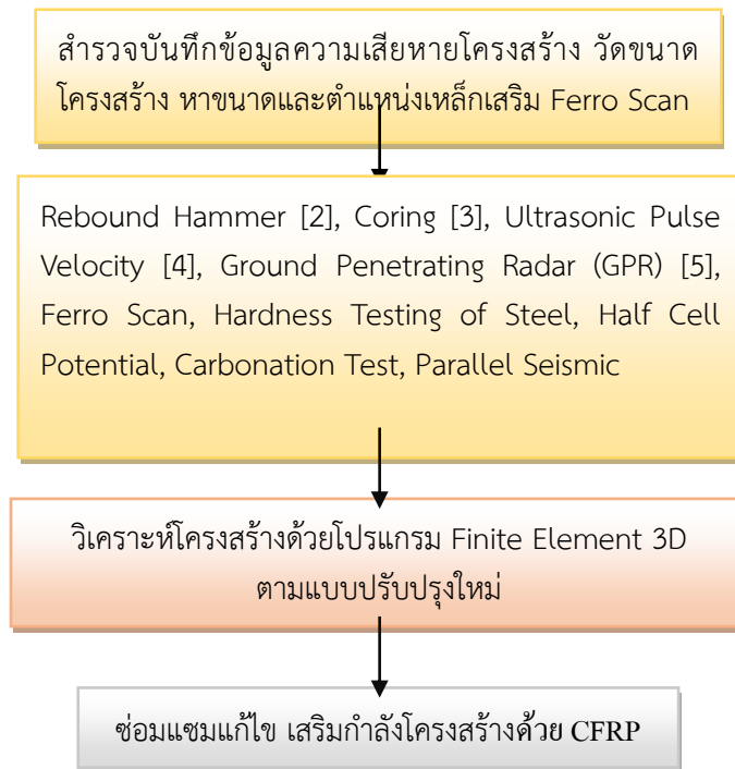
รูปที่ 2 แผนภาพแสดงขั้นตอนการตรวจสอบและเสริมกำลังโครงสร้าง [6]
