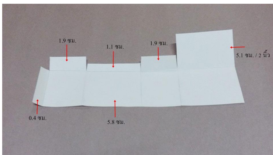
รูปที่ 4.1 ขนาดของกล่องแบบที่ 1 กระดาษสีธรรมชาติ
